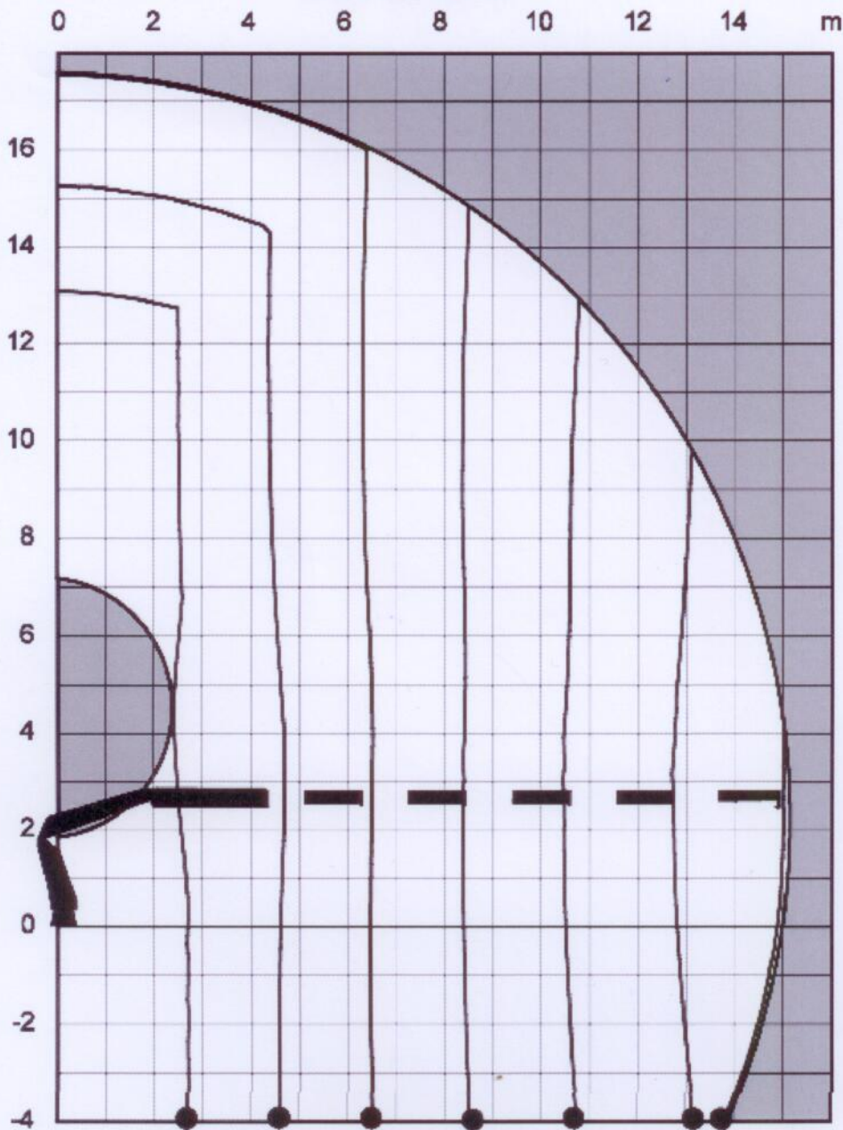
Belastungsdiagramm
